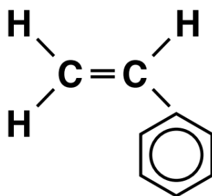
Styrene monomer
